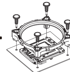
Socket 775
