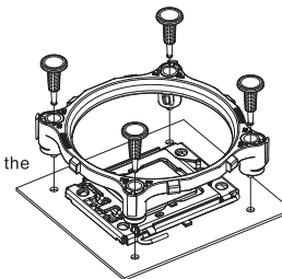
Socket 775
